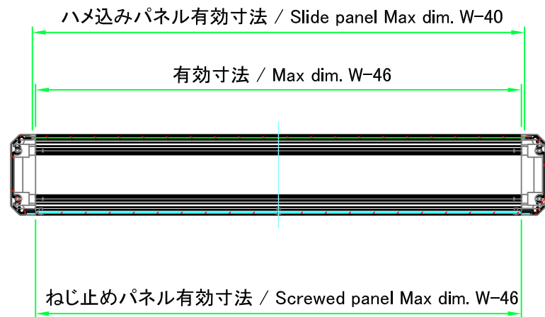
A-A (1:5)
